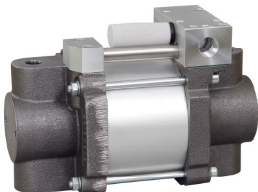
S15D двойного действия, один поршень привода воздуха
