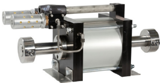
GPD60 двойного действия, один поршень привода воздуха
