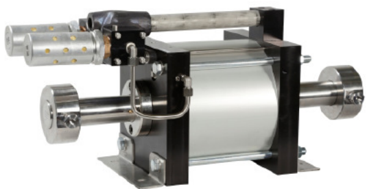
GPD120 двойного действия, один поршень привода воздуха
