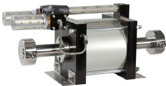
GPD260 двойного действия, один поршень привода воздуха
