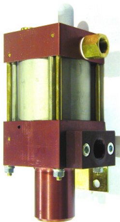
МО8 одинарного действия, один поршень привода (Стандарт = Вход Снизу)
