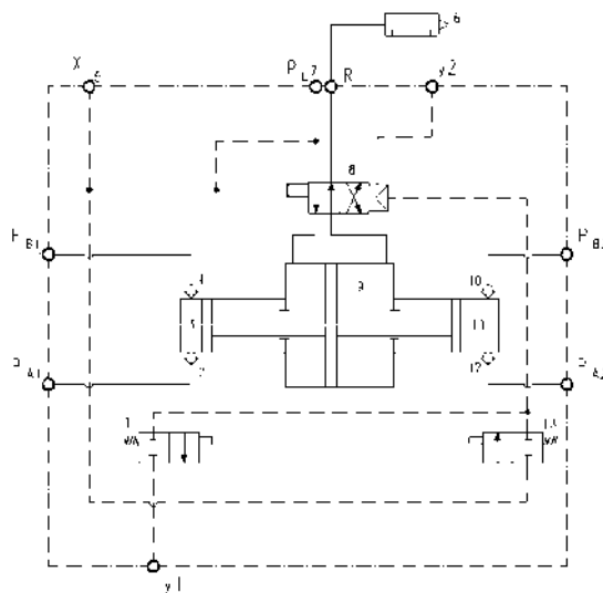
Рис. Схема соединения компрессора двойного действия
